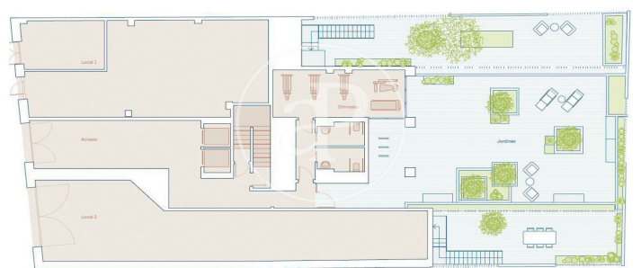
PLANTA DE ACCESO VIVIENDAS JARDIN Y ZONAS COMUNES
